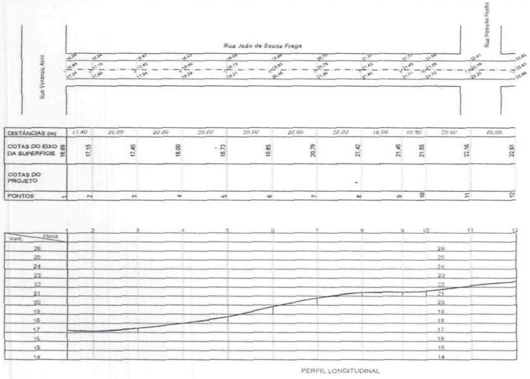
PERFIL LONGITUDINAL
