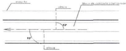
inclinação placa suspensa
