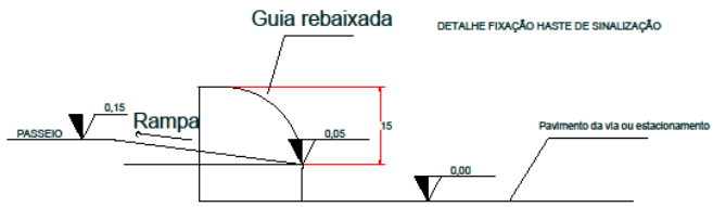
DETALHE REBAIXO MEIO FIO GARAGEM
