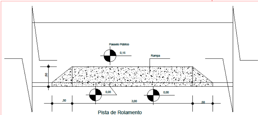
DETALHE REBAIXO MEIO FIO GARAGEM
