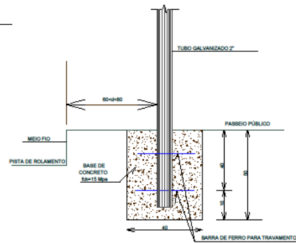
DETALHE FIXAÇÃO HASTE DE SINALIZAÇÃO
