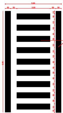
DETALHE FAIXA DE PEDESTRE
