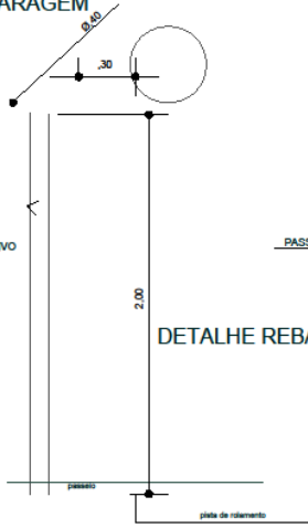
DETALHE FIXAÇÃO PLACA NO PASSEIO
