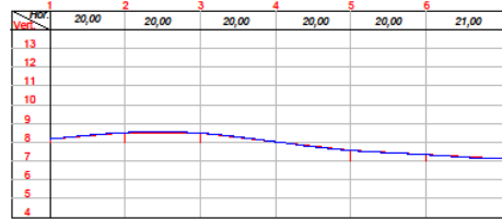
PERFIL LONGITUDINAL
